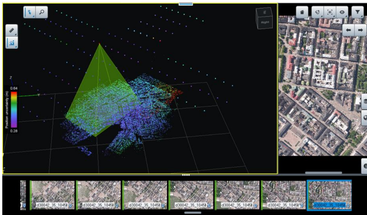
图44：显示“3D视图”选项卡中的空中三角测量计算结果示例
