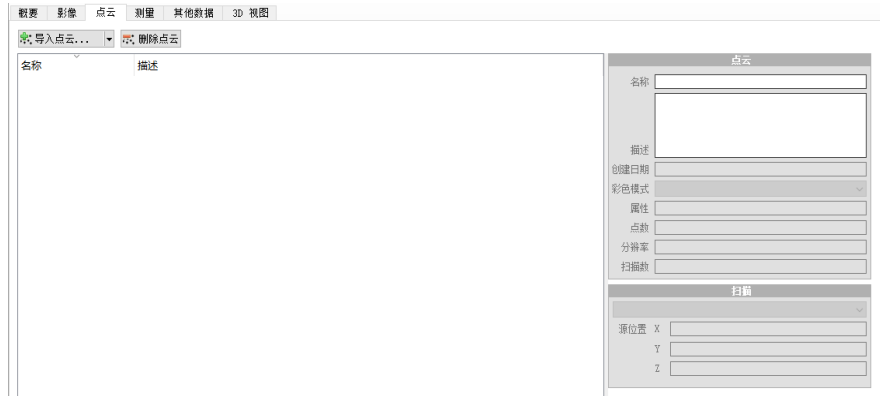
图26：“点云”选项卡
