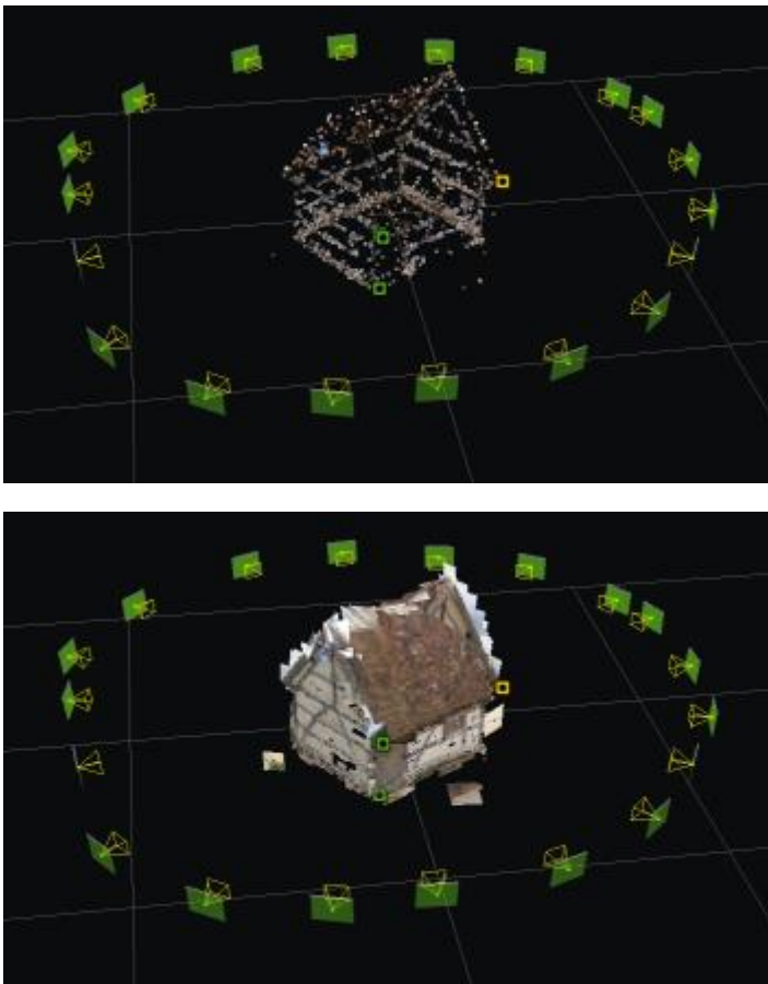
图37: 生成的连接点和相应的拼板表示
