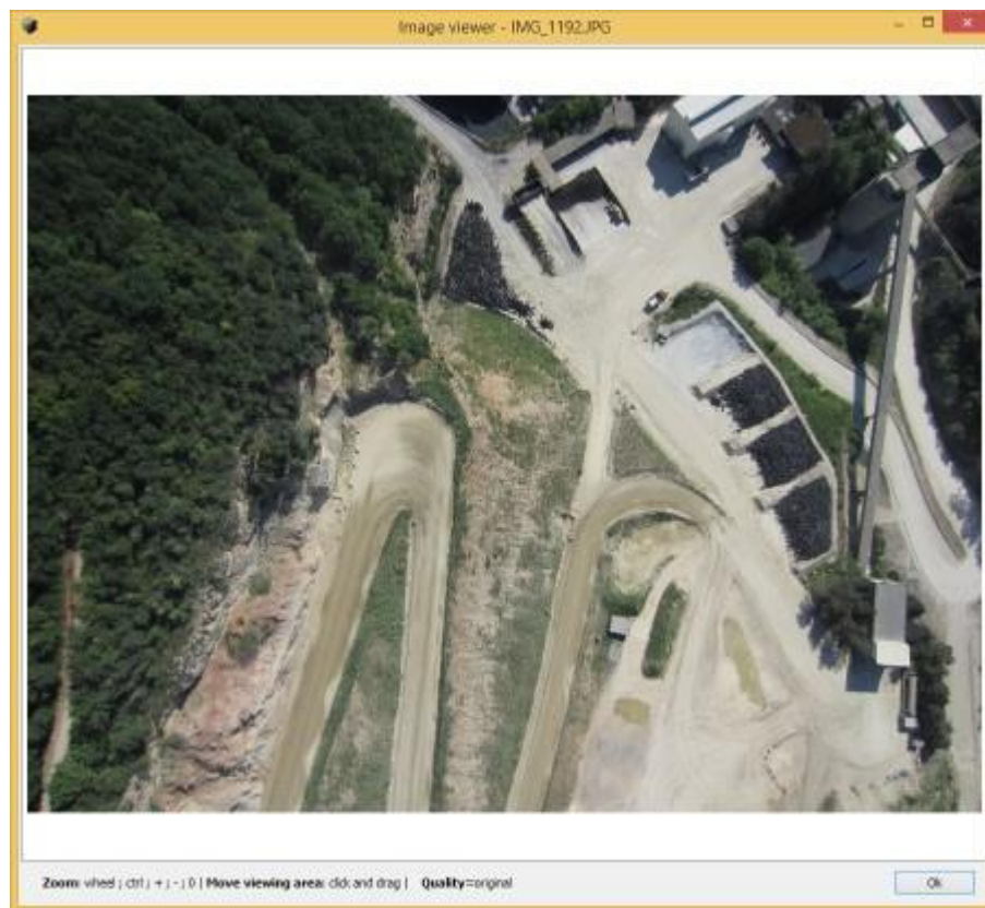
图23: 影像查看器
